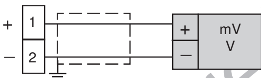
Fig. 7- V / mV input wiring
