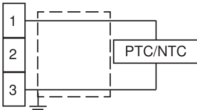
Fig. 6- PTC / NTC input wiring
